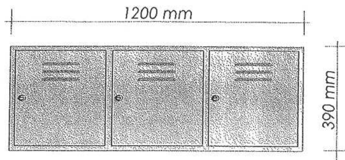
Elölnézet
